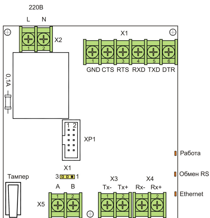
Рисунок 5 - Вид на плату БПДД-Е
