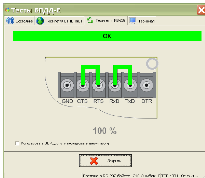
Рисунок 32 - Тестирование RS-232
