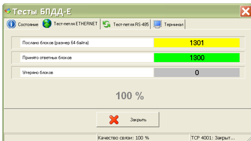
Рисунок 36 - Вкладка «Тест-петля ETHERNET»
