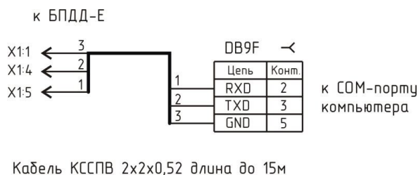
Рисунок 13 - Соединительный кабель «БПДД-Е - компьютер»
