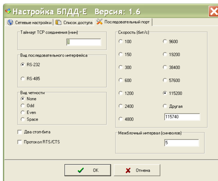
Рисунок 23 - Окно настройки последовательного порта
