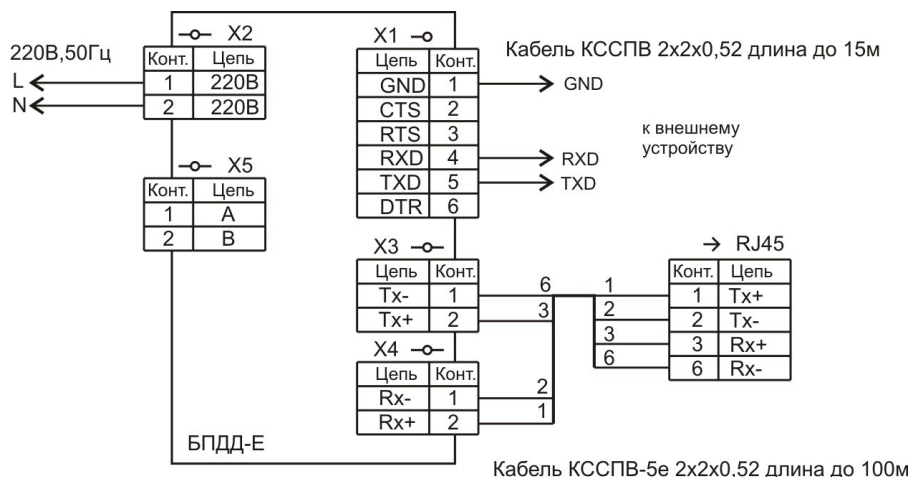
Рисунок 7 - Электрическая схема подключения БПДД-Е к внешнему устройству с интерфейсом RS-232
