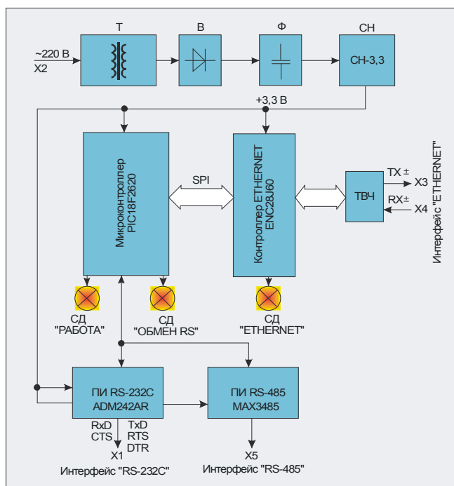
Рисунок 3 - Функциональная схема БПД-Е
