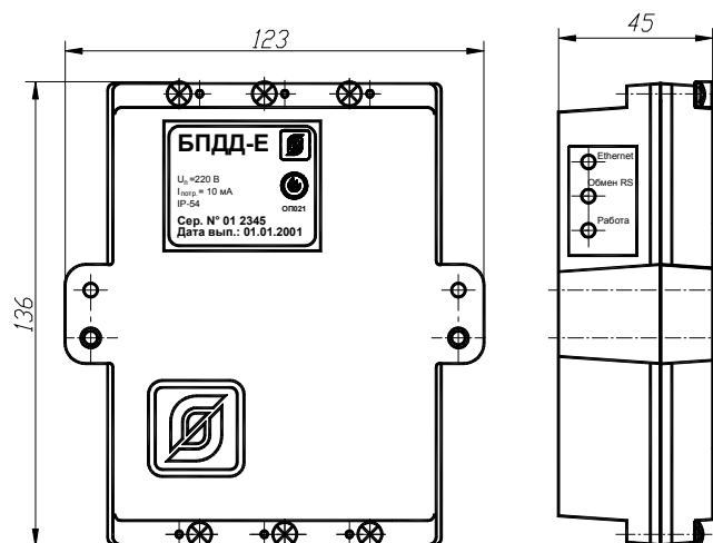
Рисунок 4 - Габаритные размеры БПДД-Е
