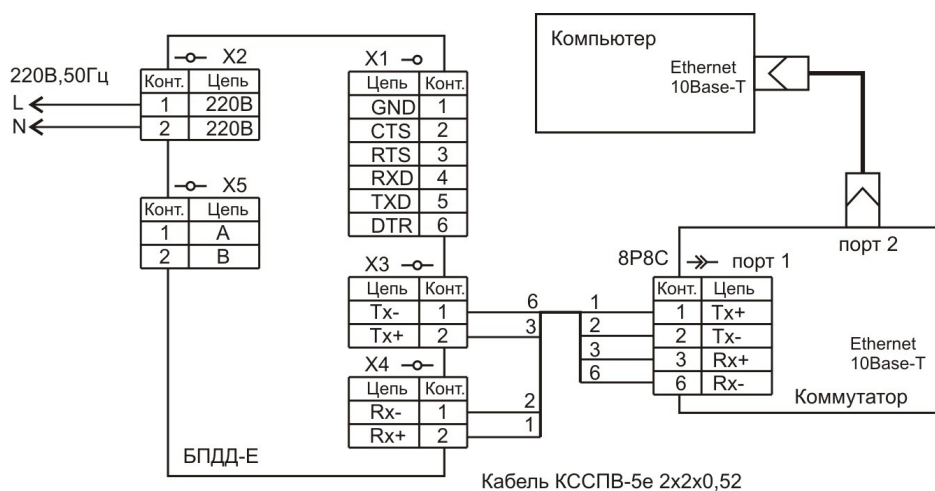
Рисунок 30 - Подключение компьютера к БПДД-Е
