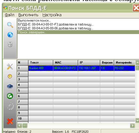
Рисунок 19 - Результаты поиска в программе RASOS
