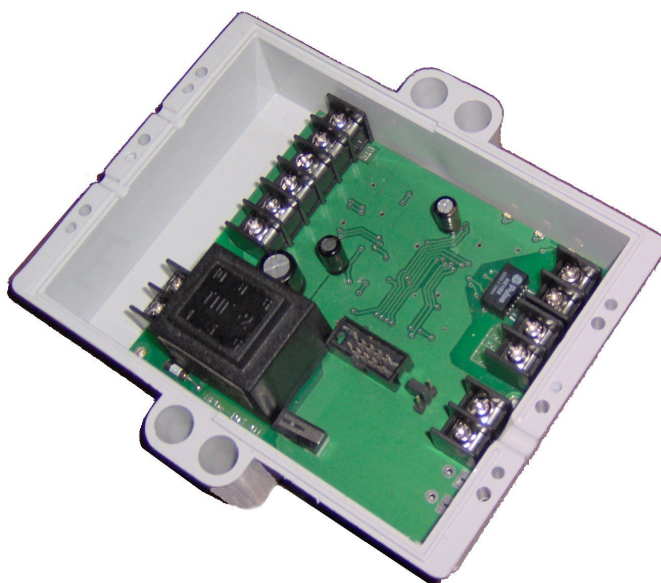
Рисунок 6 - БПДД-Е (крышка снята)
