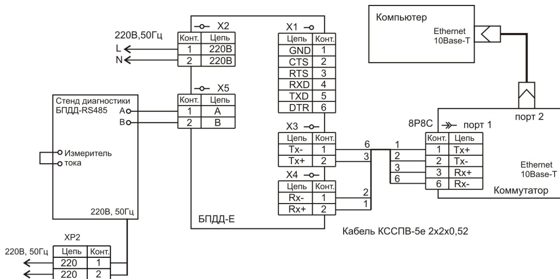
Рисунок 33 - Схема контроля работоспособности интерфейса RS-485
