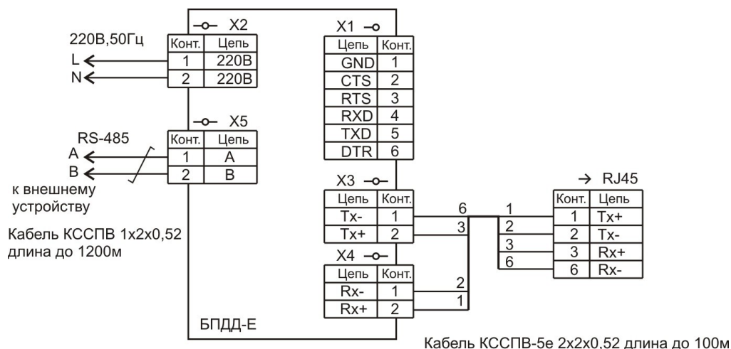
Рисунок 8 - Электрическая схема подключения БПДД-Е к внешнему устройству с интерфейсом RS-485
