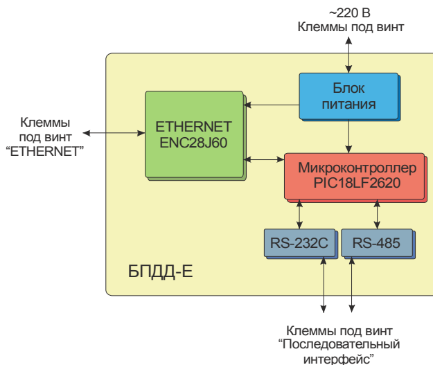
Рисунок 2- Общая структурная схема БПДД-Е
