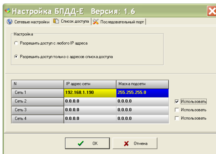
Рисунок 22 – Изменение списка доступа
